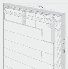
Horizontale Verlegung
