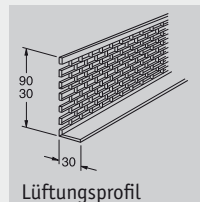
Lüftungsprofil
