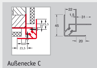
Alu-Außeneckprofil
