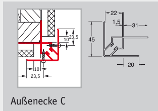
Alu-Außeneckprofil
