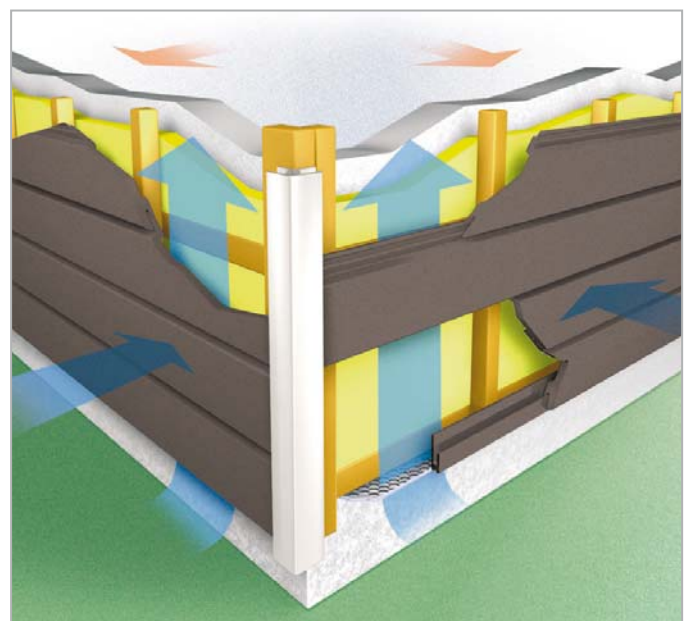
WERZALIT Fassadensysteme schützen als vorgehängte, hinterlüftete Fassade nachhaltig das Bauwerk.
